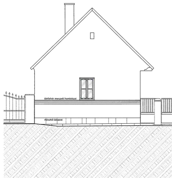
Délnyugati homlokzat
