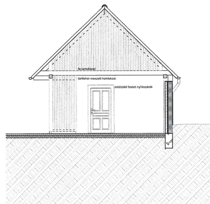
Északkeleti homlokzat
