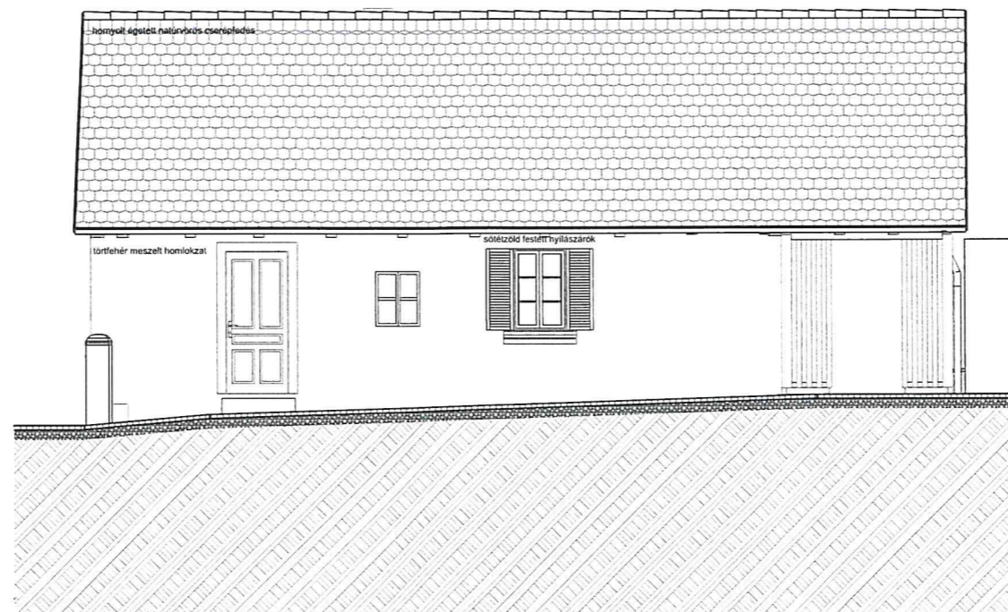
Délkeleti homlokzat
