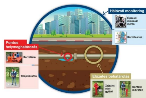
2. ábra – Az aktív szivárgáskeresés tevékenység főbb lépései
