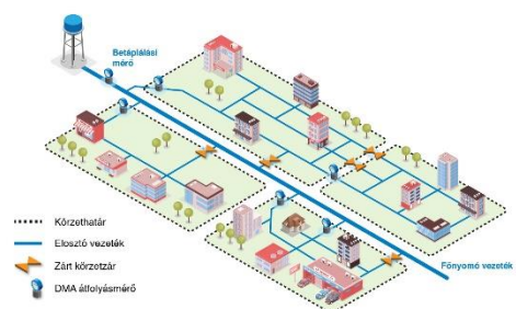
3. ábra – DMA körzet sémája
