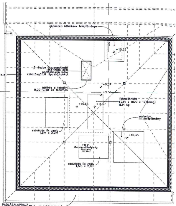
PADLÁSLAPRAJZ 30 - os tetőszerkezeti M = 1 : 50
